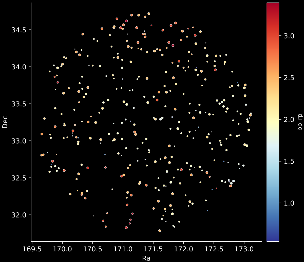
APOGEE DR17 Field: [169-08] Stars: 369
