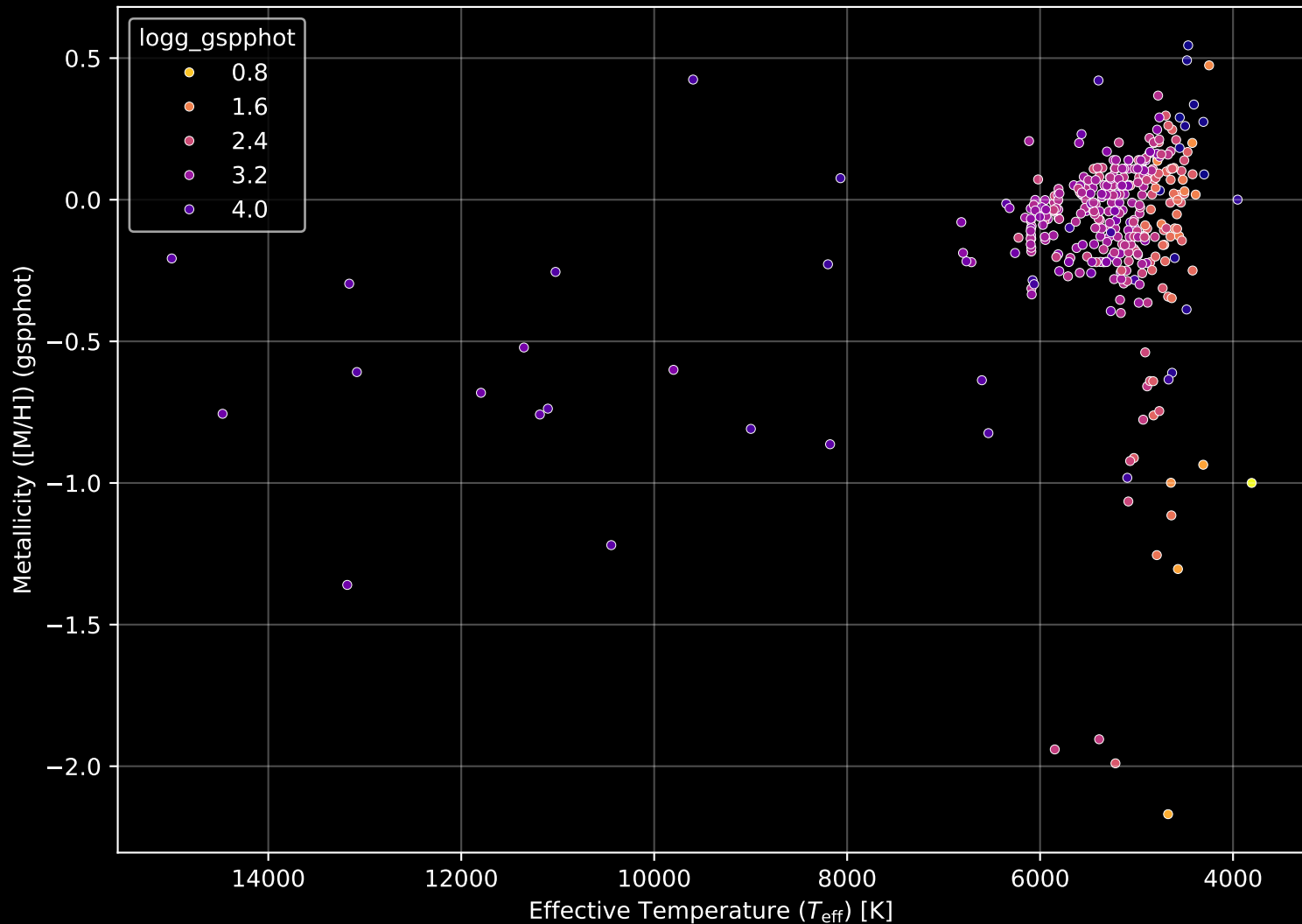
APOGEE DR17 Field: [169-08] Stellar Population Parameters (n= 369)
